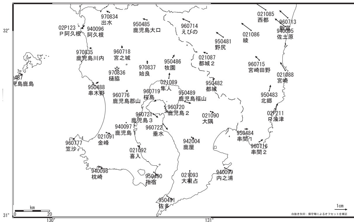
桜島周辺の地殻変動（水平）
