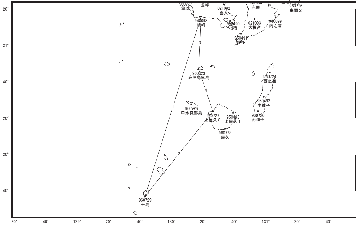
諏訪之瀬島・薩摩硫黄島周辺 GNSS連続観測基線図
