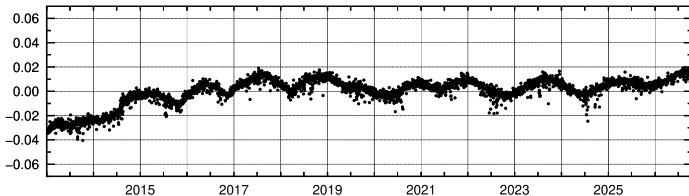
(m) (3) 大島 1 (93051)-大島 3 (960594) 斜距離
