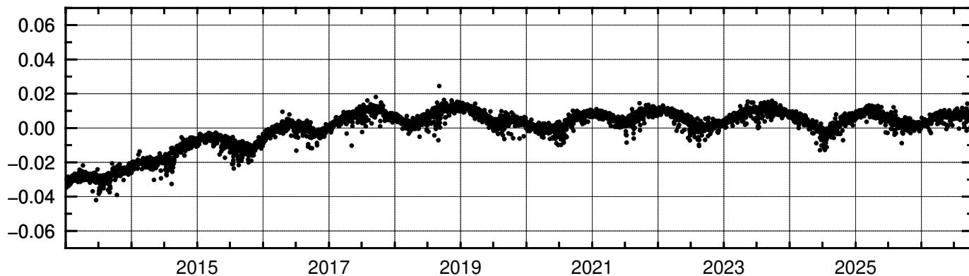
(m) (4) 大島 3 (960594)-大島 2 (93055) 斜距離
