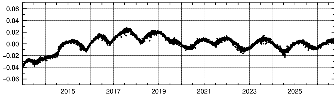
(m) (1) 大島 1 (93051)-大島 2 (93055) 斜距離
