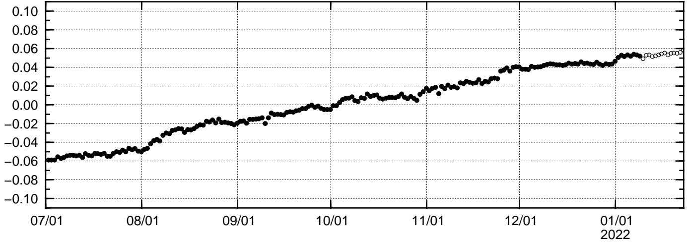
(m) (6) 硫黄島 1 (960604) - M硫黄島 A (149086) 東西
