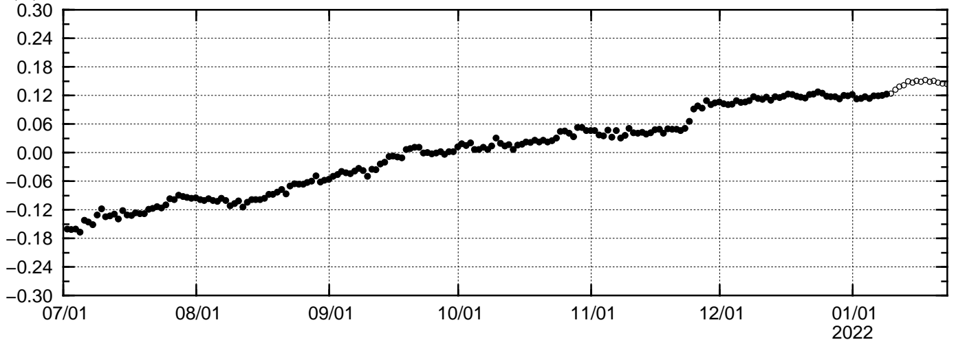
(m) (6) 硫黄島 1 (960604) - M硫黄島 A (149086) 比高
