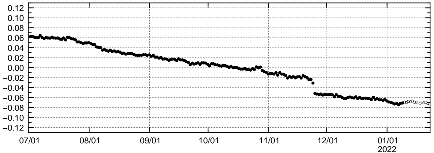
(m) (6) 硫黄島 1 (960604) - M硫黄島 A (149086) 南北
